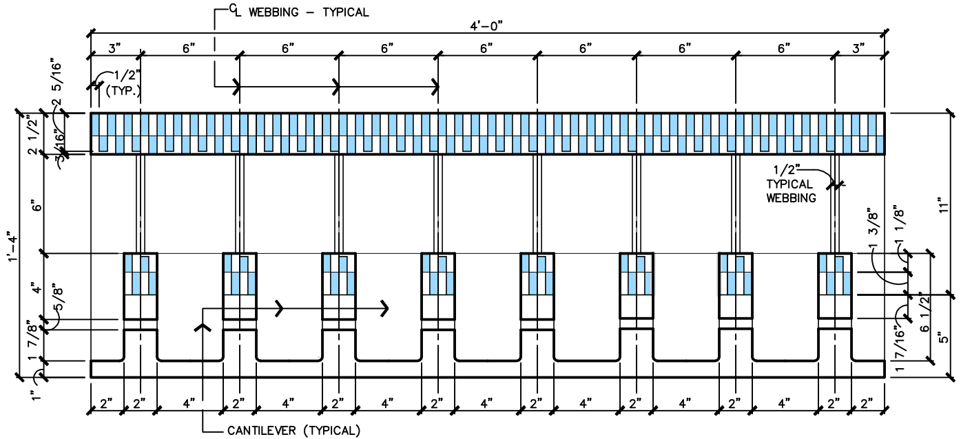
2 TOP VIEW 05a SCALE: 1 1/2" = 1'-0"
