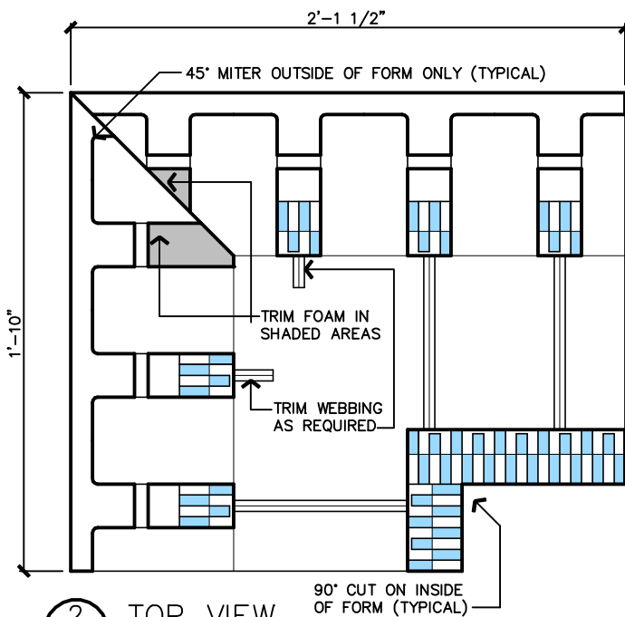
2 TOP VIEW SCALE: 1 1/2" = 1'-0"
