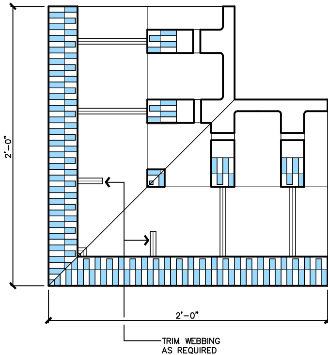
1 44a TOP VIEW SCALE: 1 1/2" = 1'-0"
